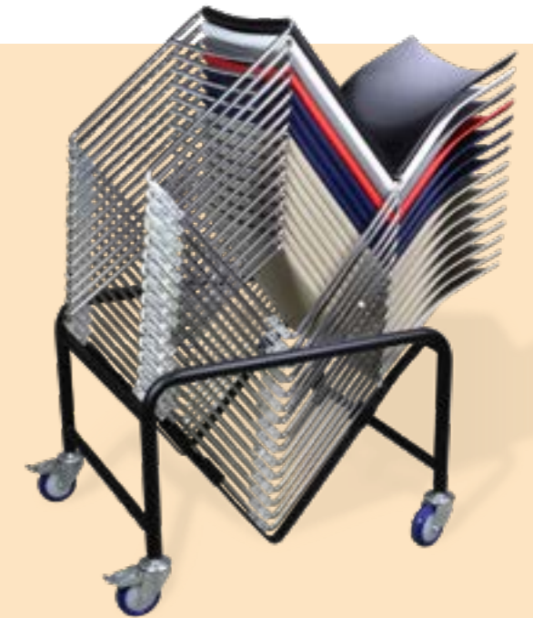
TROLLEY 3522 Transportwagen für Kufenstühle, bis 40 Stück
